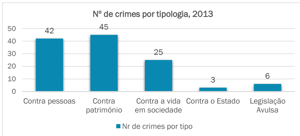
Gráfico 61 – Nº de crimes registados por tipologia de crime, 2013. - Fonte: Pordata, 2013
