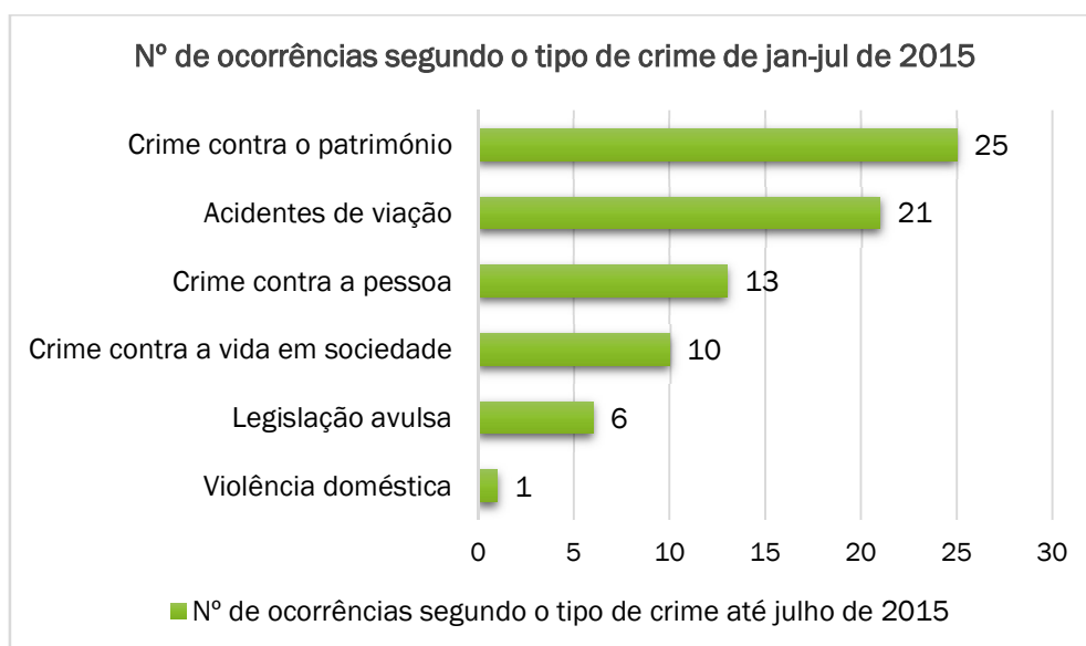
Gráfico 62- Número de ocorrências segundo o tipo de crime no último ano (até julho de 2015) na GBR de Fornos de Algodres. - Fonte: GNR de Fornos de Algodres
