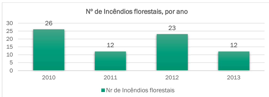
Gráfico 63 – Nº de Incêndios Florestais por ano. - Fonte: Pordata
